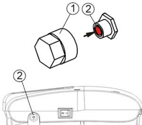
Obr. 29: Havarijní termostat
