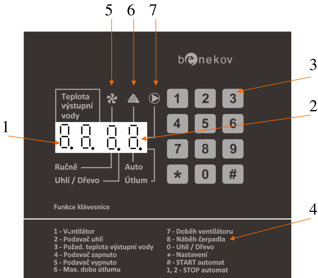
Obr. č. 1 Čelní panel regulátoru RKU1.5
