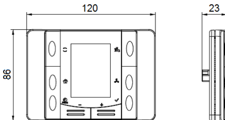
Obr. č. 1 Základní rozměry prostorového přístroje POL 822.70
