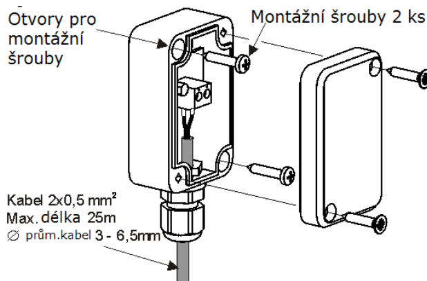
Obr. 20 Připojení venkovního čidla CT6-P
