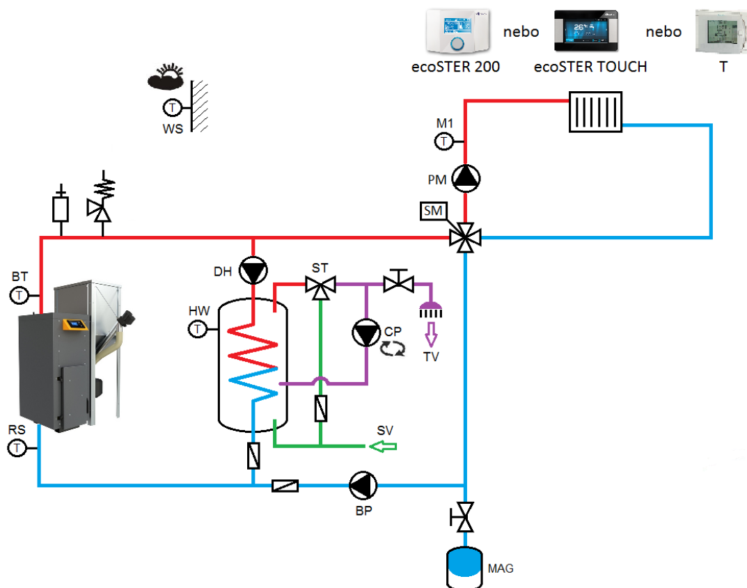
Obr. 13 Doporučené hydraulické schéma bez akumulární nádrže
