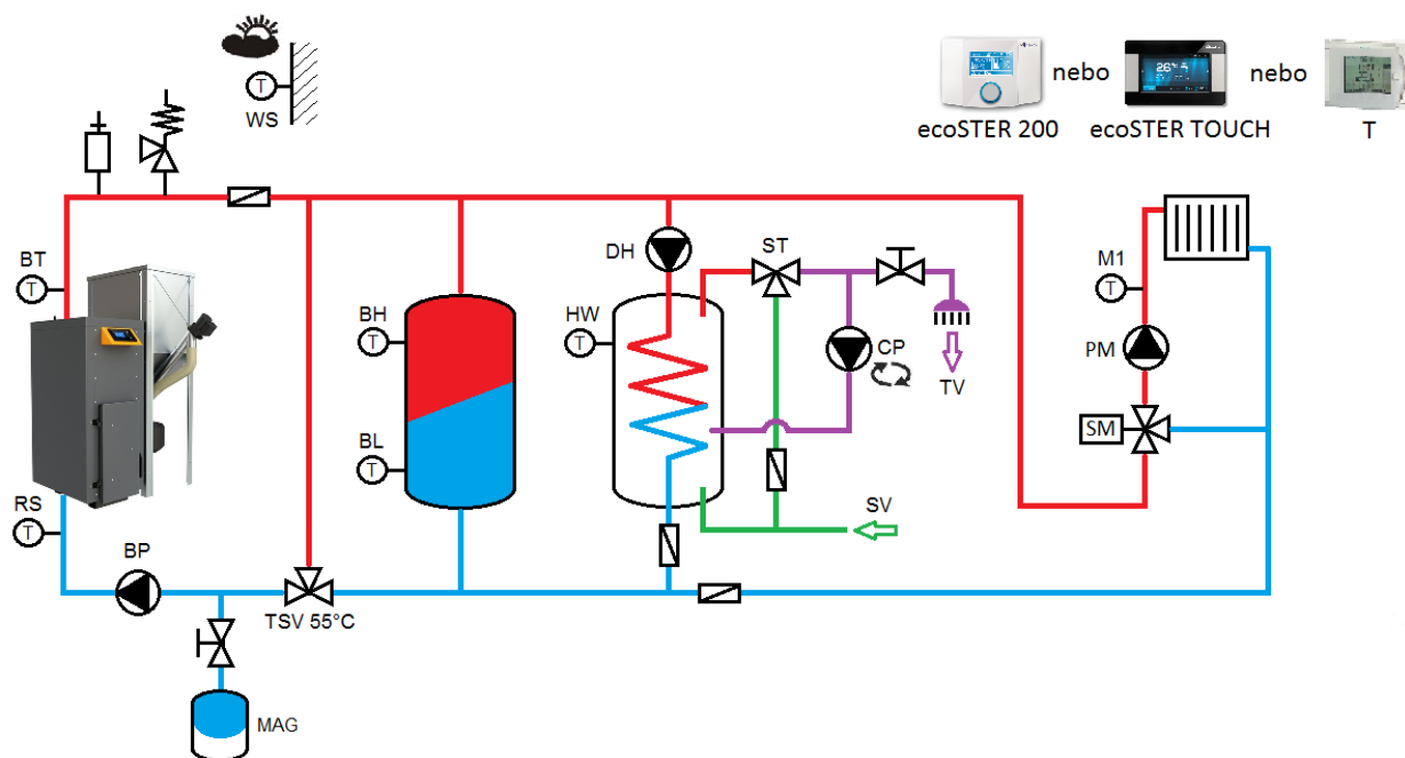
Obr. 14 Doporučené hydraulické schéma s akumulční nádrží
