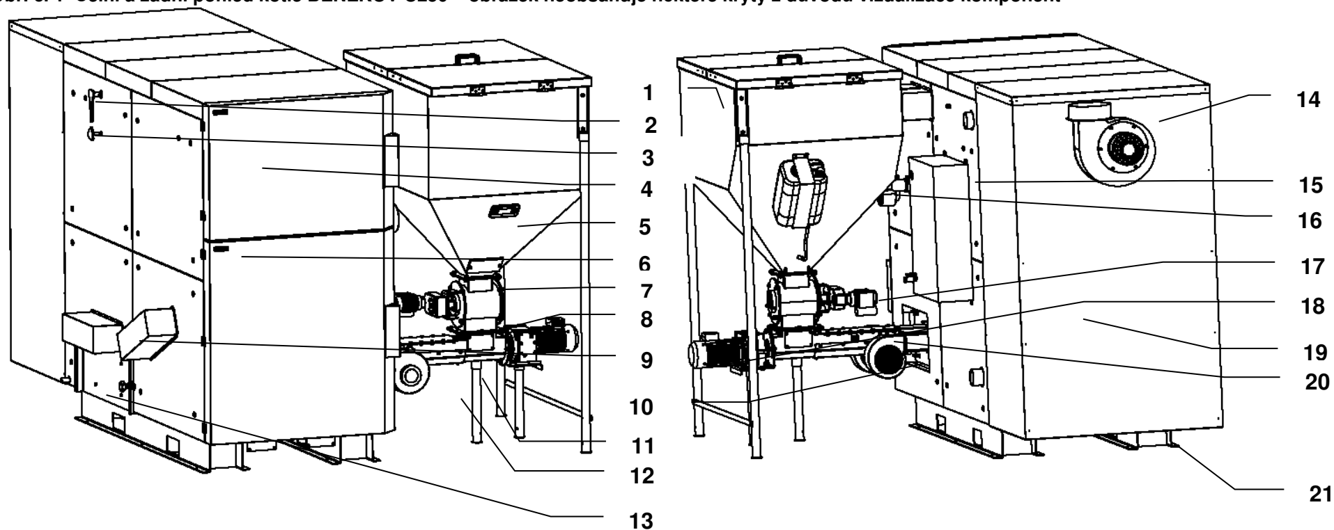
Obr. č. 1 Čelní a zadní pohled kotle BENEKOV C250 – obrázek neobsahuje některé kryty z důvodů vizualizace komponent
