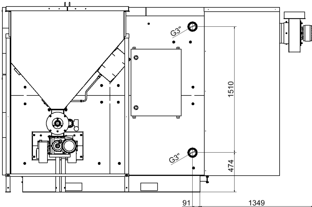
Obr. č. 6 Připojovací rozměry kotle BENEKOV C250 na topný systém
