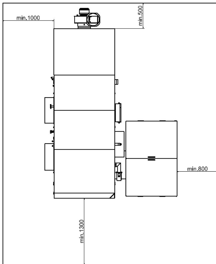
Obr. č. 3 Umístění kotle v kotelně
