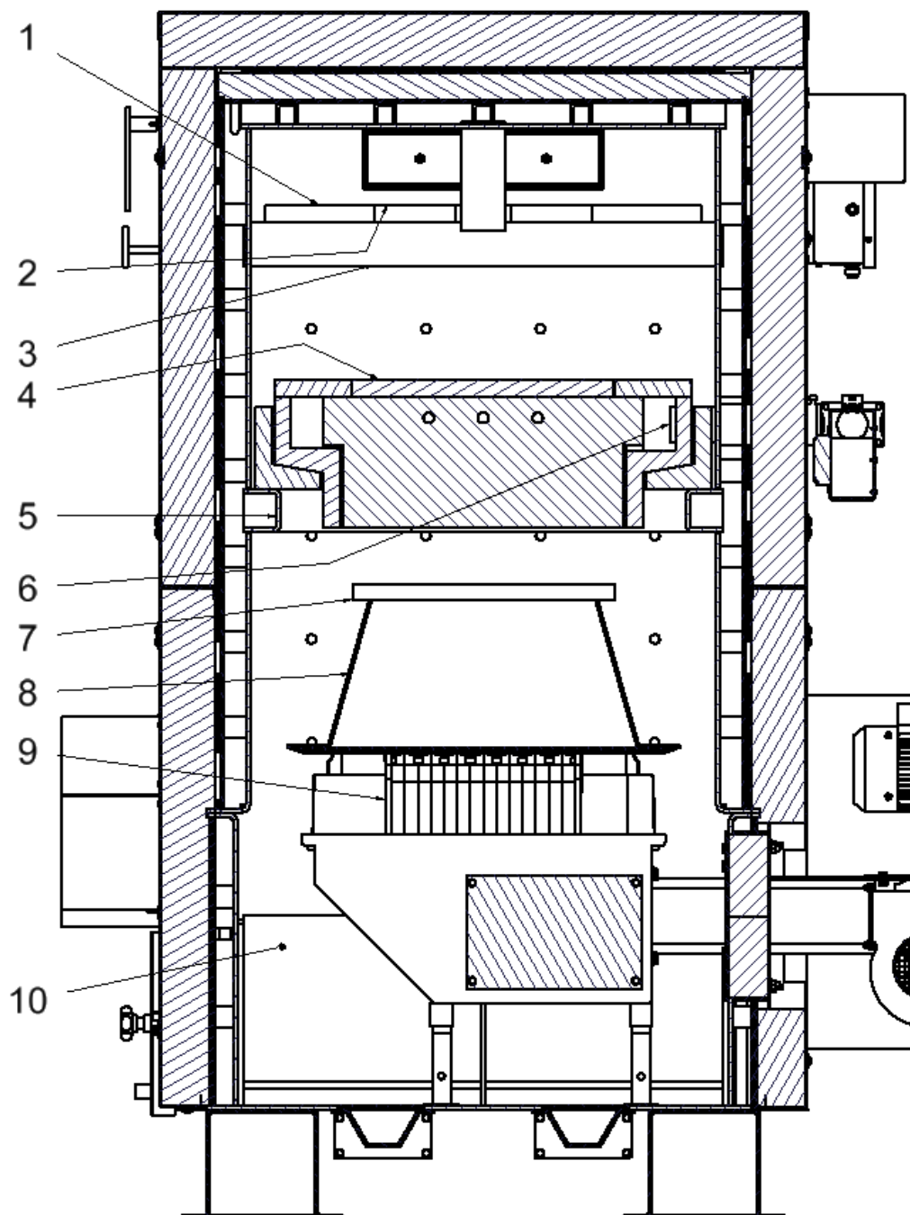
Obr. č. 7 Řez spalovací komorou kotle
