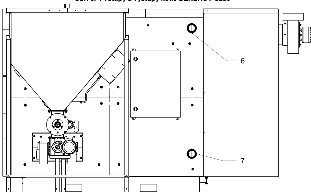
Obr. č. 4 Vstupy a výstupy kotle BENEKOV C250
