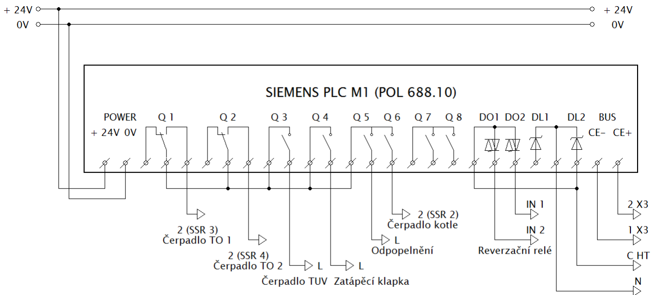
EI. schéma vstupů POL 985
