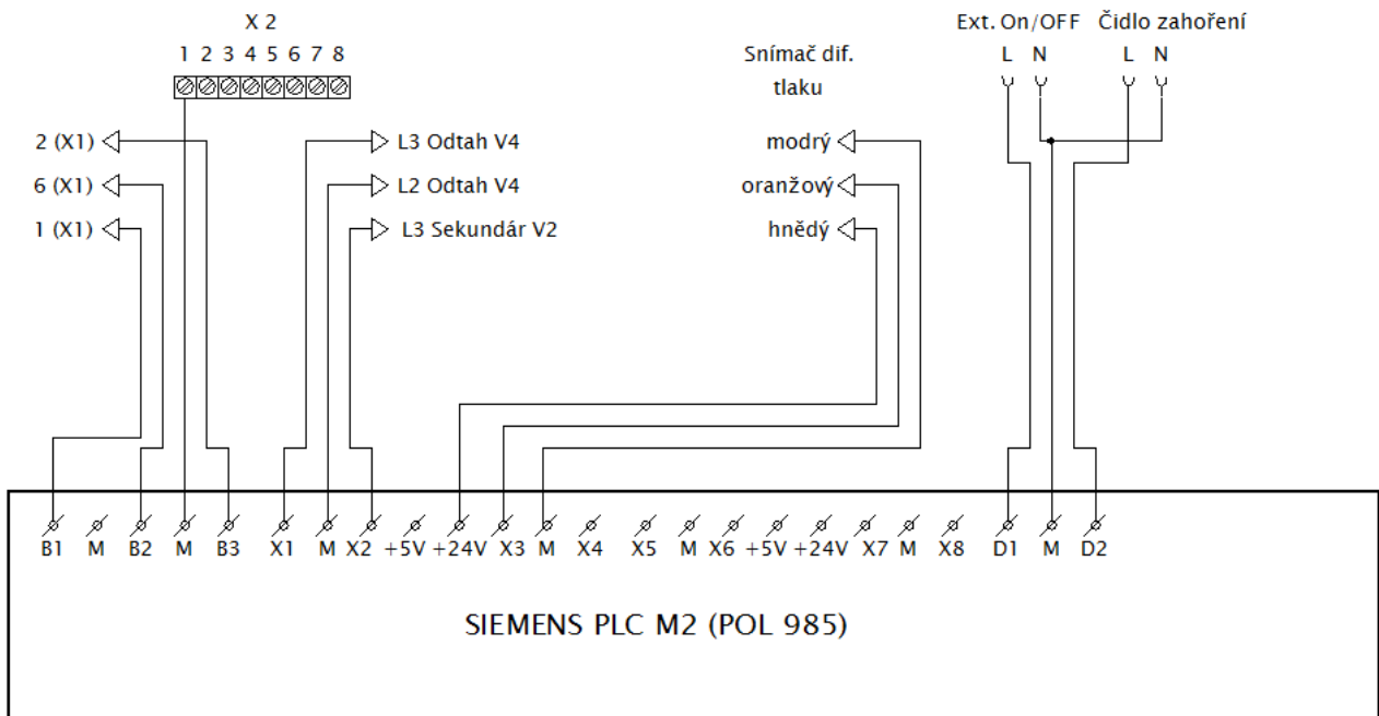
EI. schéma výstupů POL 985
