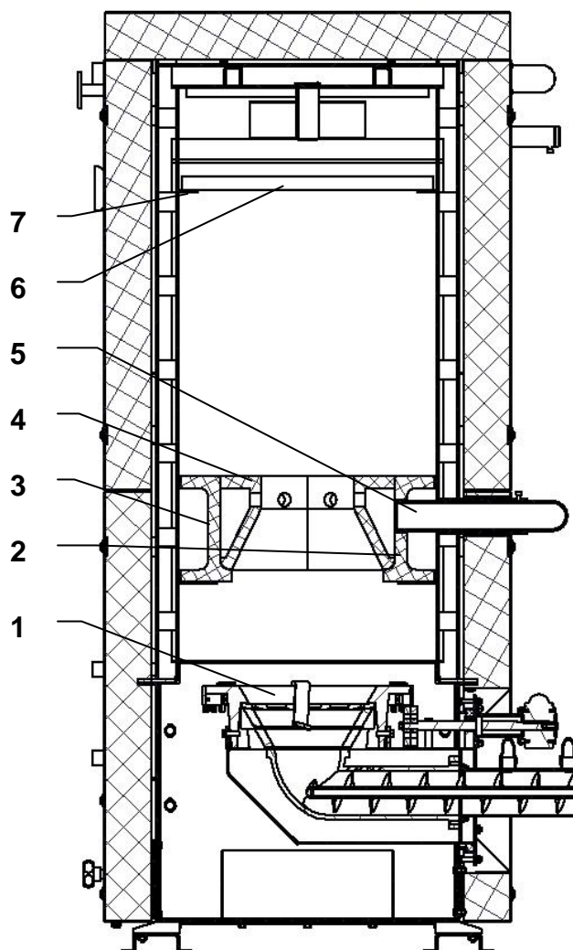
Obr. č. 7 Řez spalovací komorou kotle
