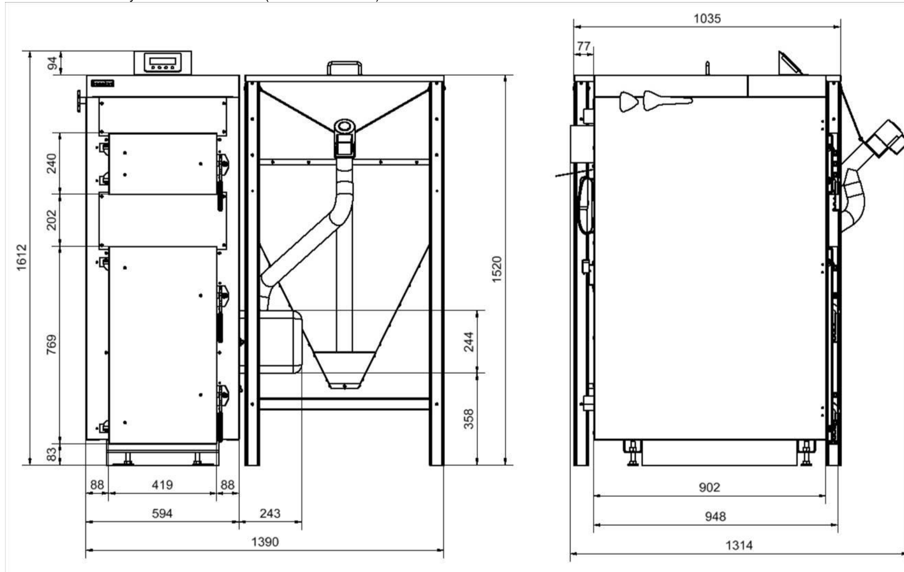
Obr. 14 Základní rozměry kotle BENEKOV K35 (verze STANDART)
