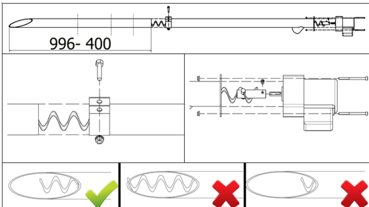
Obr. 35 Schéma podavače VENMA
