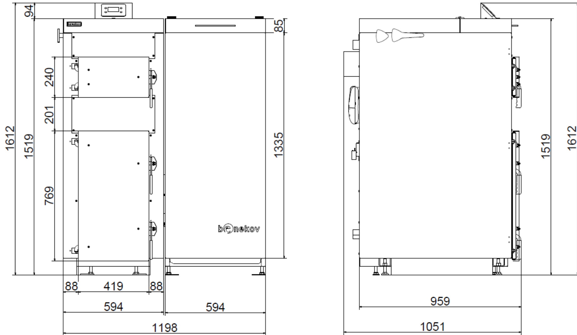
Obr. 16 Základní rozměry kotle BENEKOV K35 (verze PLUS)
