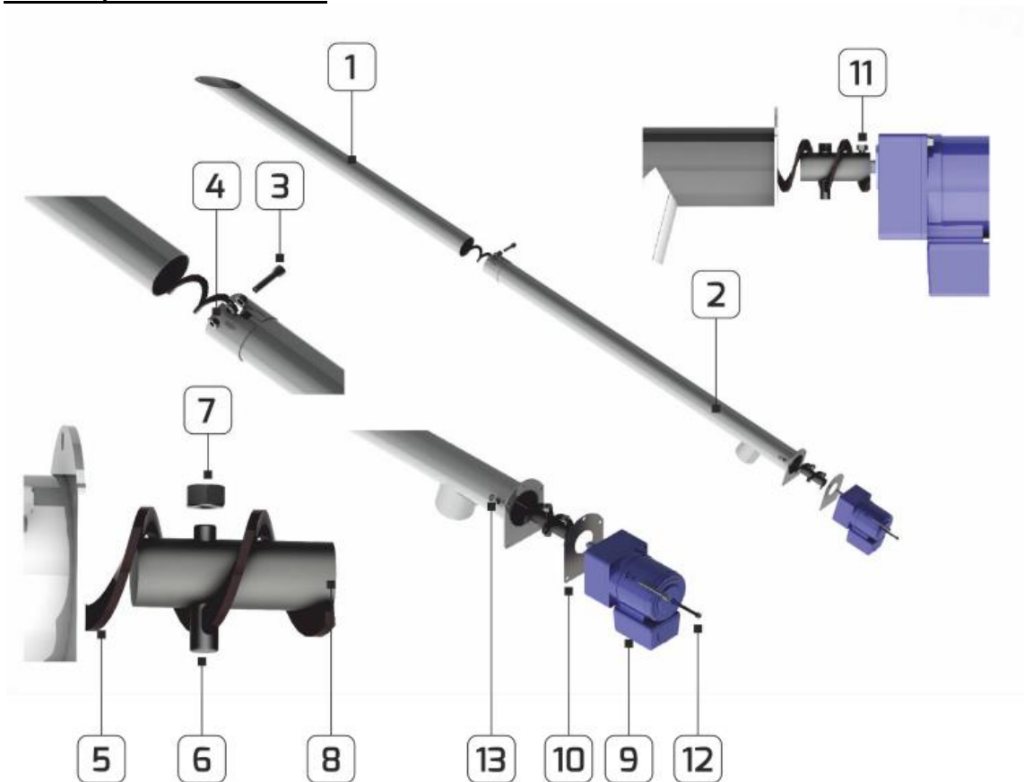
Obr. 29 Schéma podavače PELLASX
