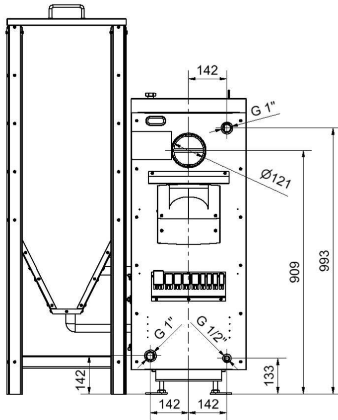
Obr. 40 Připojovací rozměry kotle BENEKOV K14
