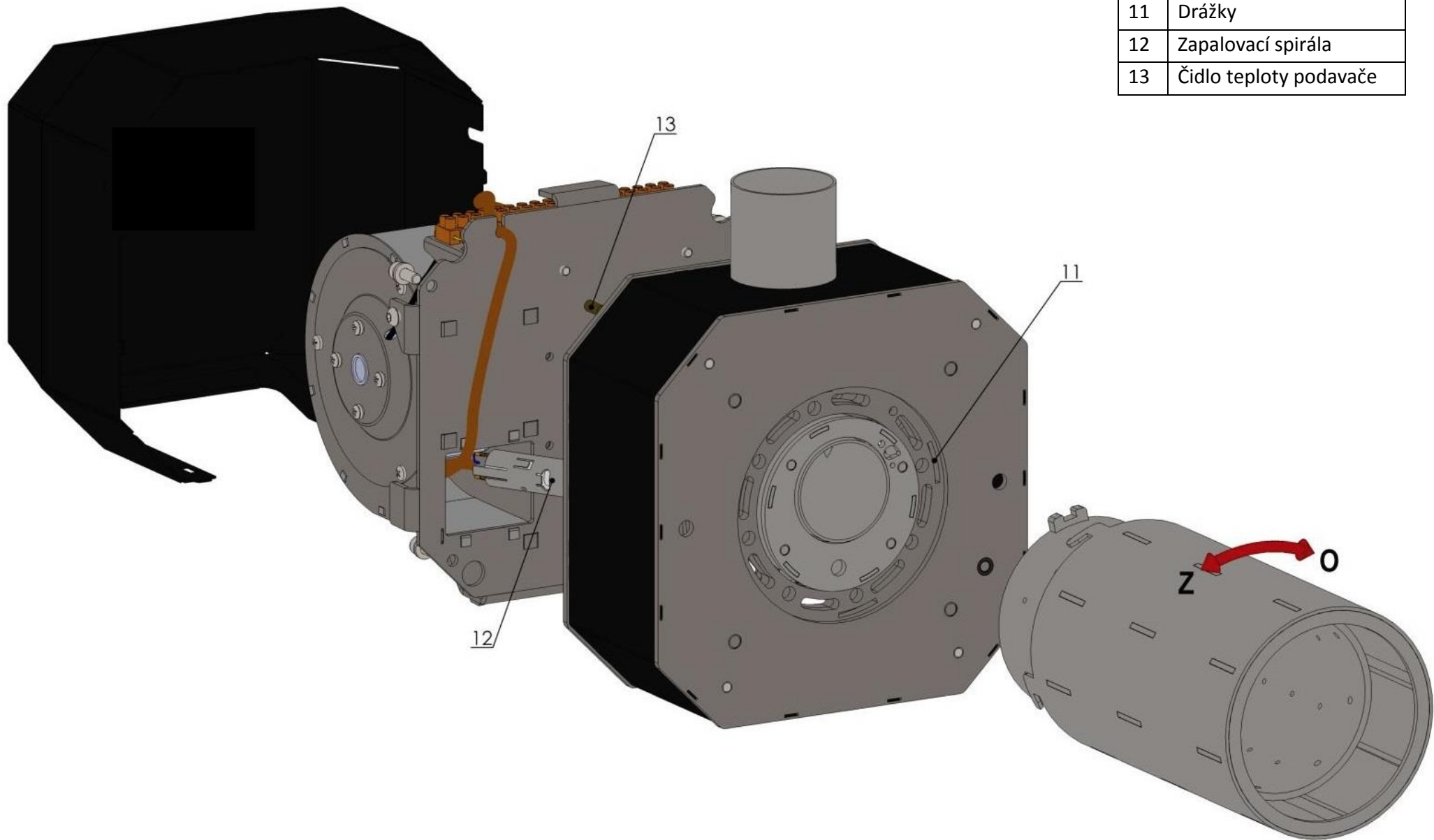
Obrázek 15. Čištění provzdušňovací komory hořáku
