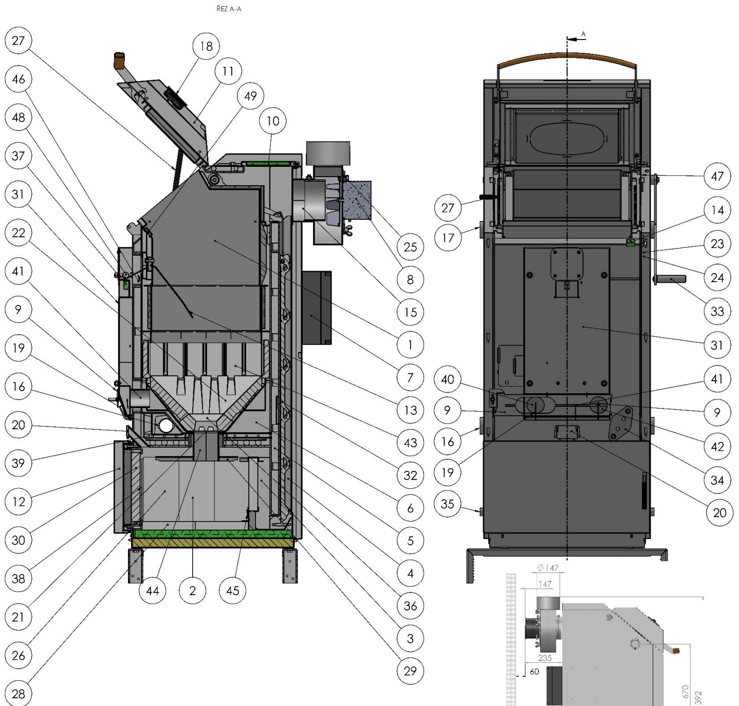
Obrázek 2. Řez kotlem DK12 a DK18
