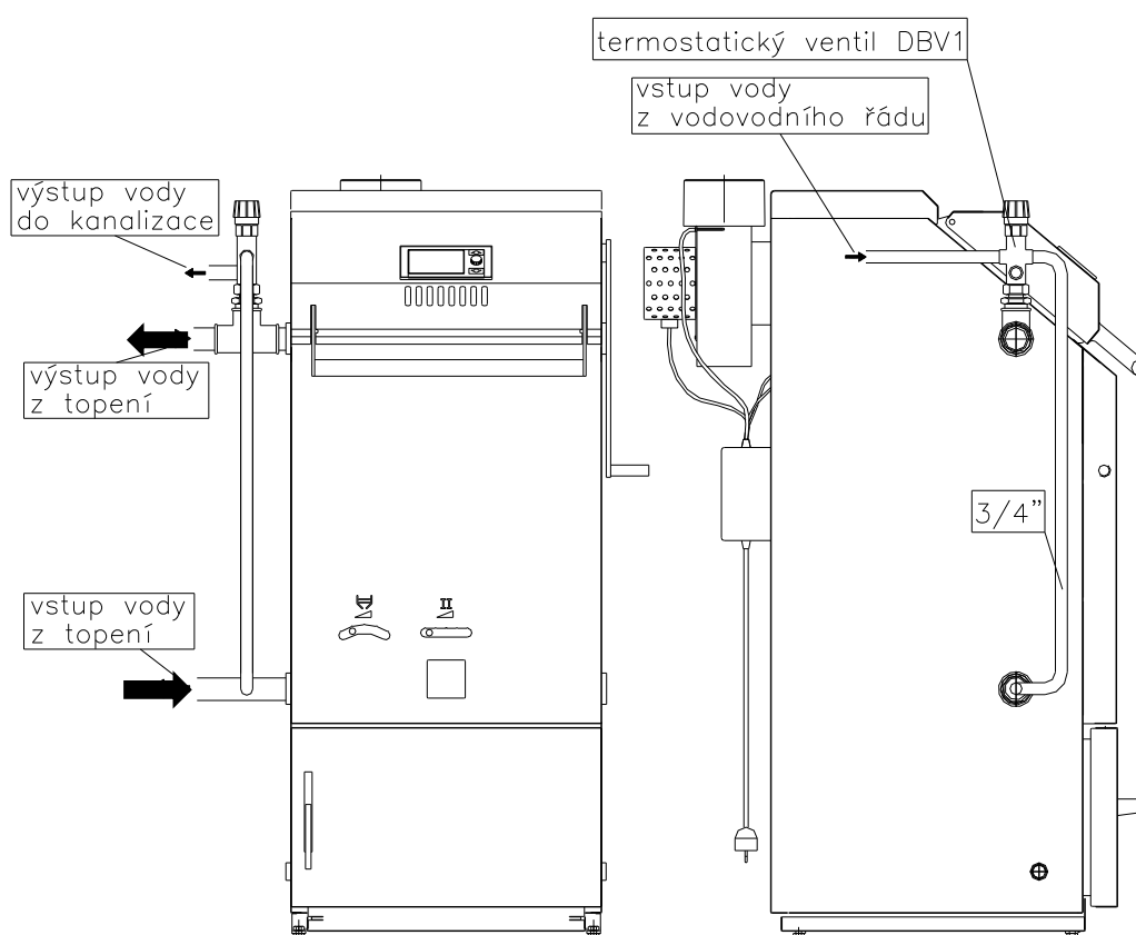
Obrázek 6. Zapojení samočinného dochlazování
