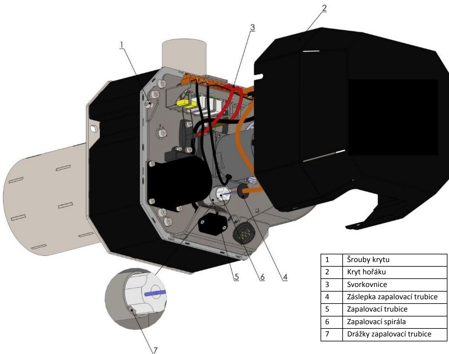
Obrázek 19. Výměna zapalovací spirály
