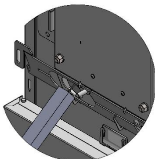
Obrázek 11. Zajištění klapky vzduchu
