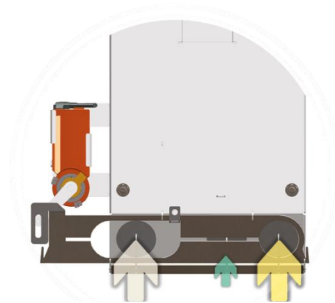
Obrázek 20. Přesuvná clona a servo pohon
